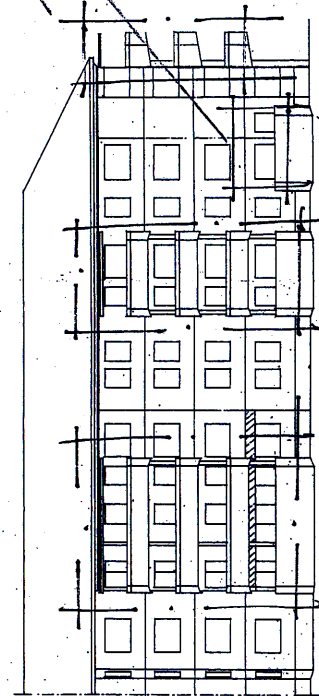
A1 GATUFASAD MOT SYD-ÖST
